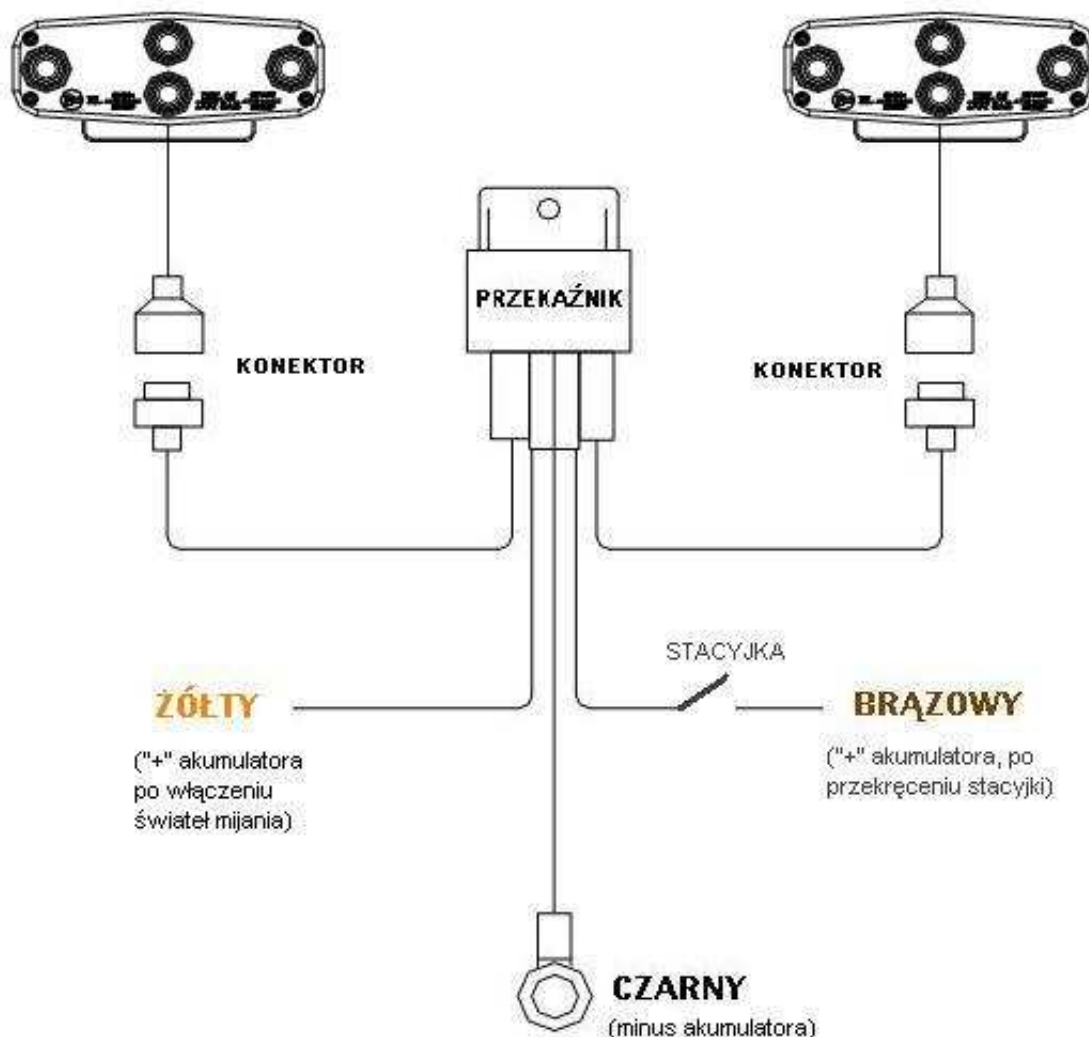
Rys. 3 Schemat połączenia MAGIC DRL 5 do instalacji samochodowej..
