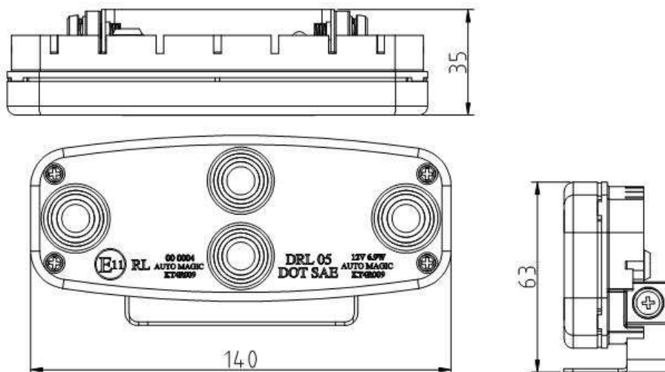
Rys. 1 Wymiary lampy MAGIC DRL 5.
