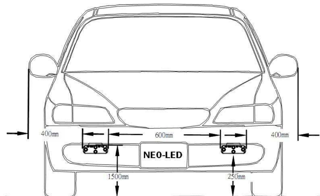
Rys. 2 Rozmieszczenie lamp.
