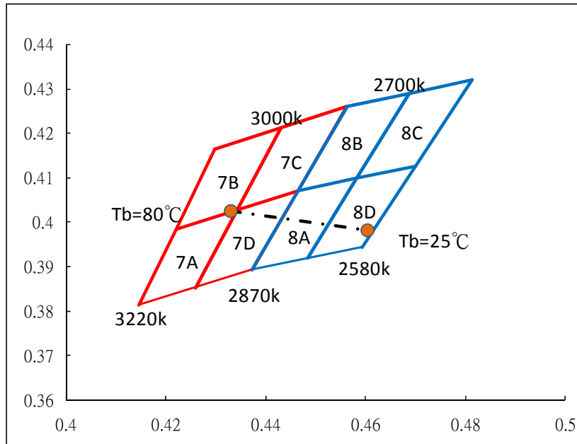
ANSI Bin Table (2580k~3220k)
